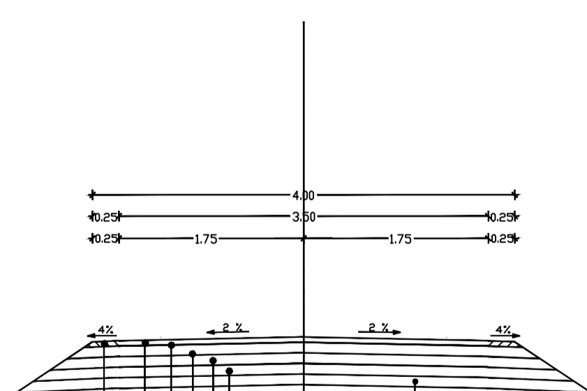
ΤΥΠΙΚΗ ΔΙΑΤΟΜΗ ΔΡΟΜΟΥ ΤΥΠΟΥ "Η1" ΚΛΙΜΑΚΑ 1/50
